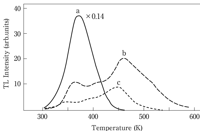
図 6 CaF 2 焼結体の TL グロー曲線
