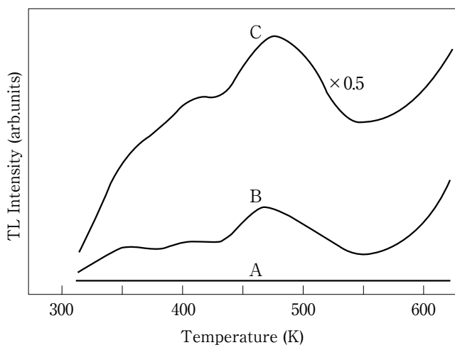
図3 蛍光灯の光（照度230lx, 約 5 \times 10^{-3} \text{J} \cdot \text{m}^{-2} \cdot \text{s}^{-1} ）に曝した \text{CaF}_2:\text{Tb} の TL グロー曲線
