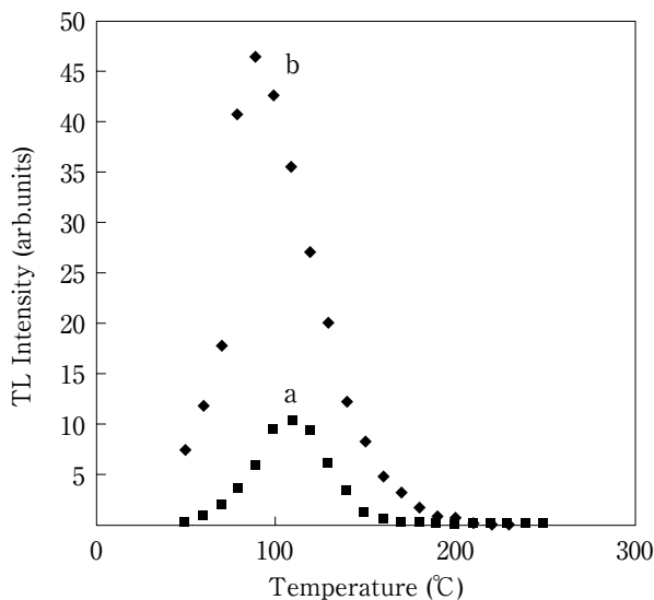
図8 TL グロー曲線
