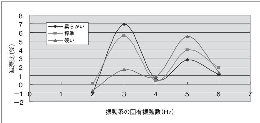
図5 正弦波掃引試験による減衰比の比較 (φ 150mm)
