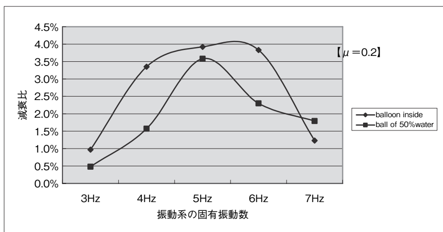
図4 正弦波加振実験結果
