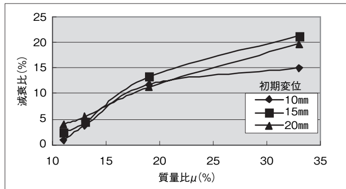
(b) 質量比の影響
