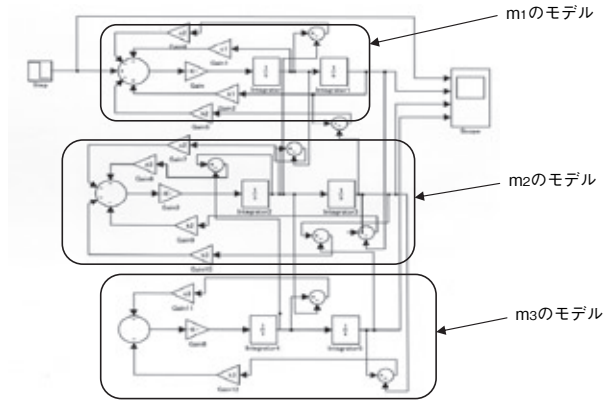
(b) SIMULINKモデル
