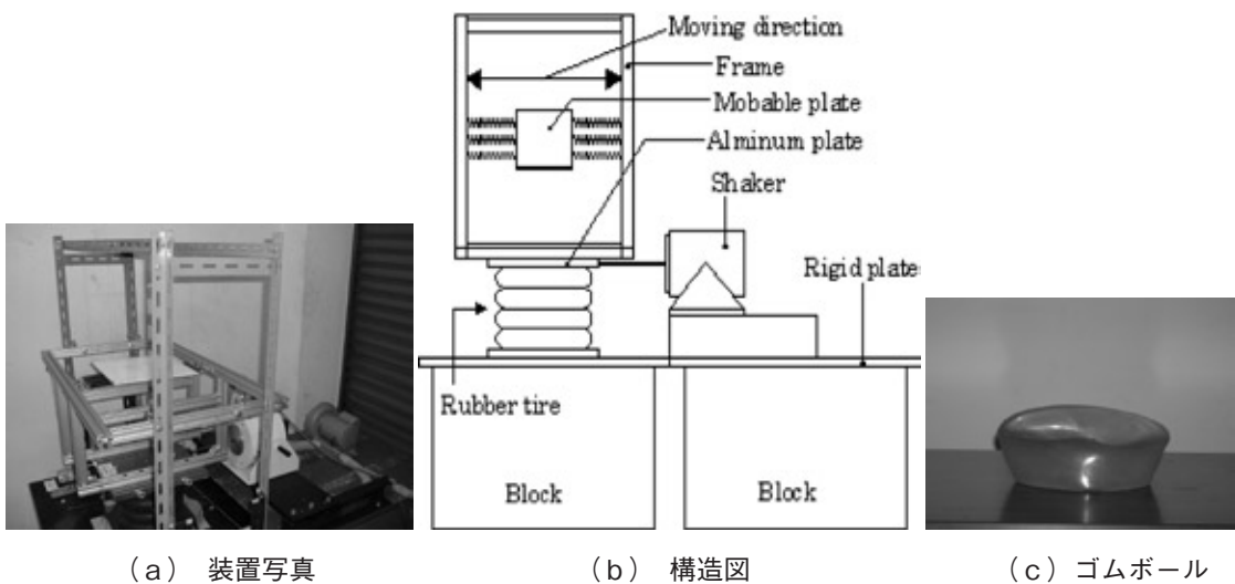
図2 実験装置
