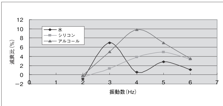
図6 内部液体の種類による減衰比の違い
