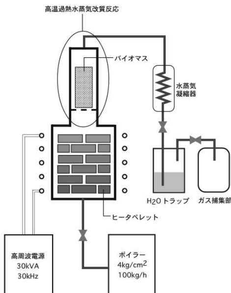
図4 高温過熱水蒸気によるバイオマス改質システム
